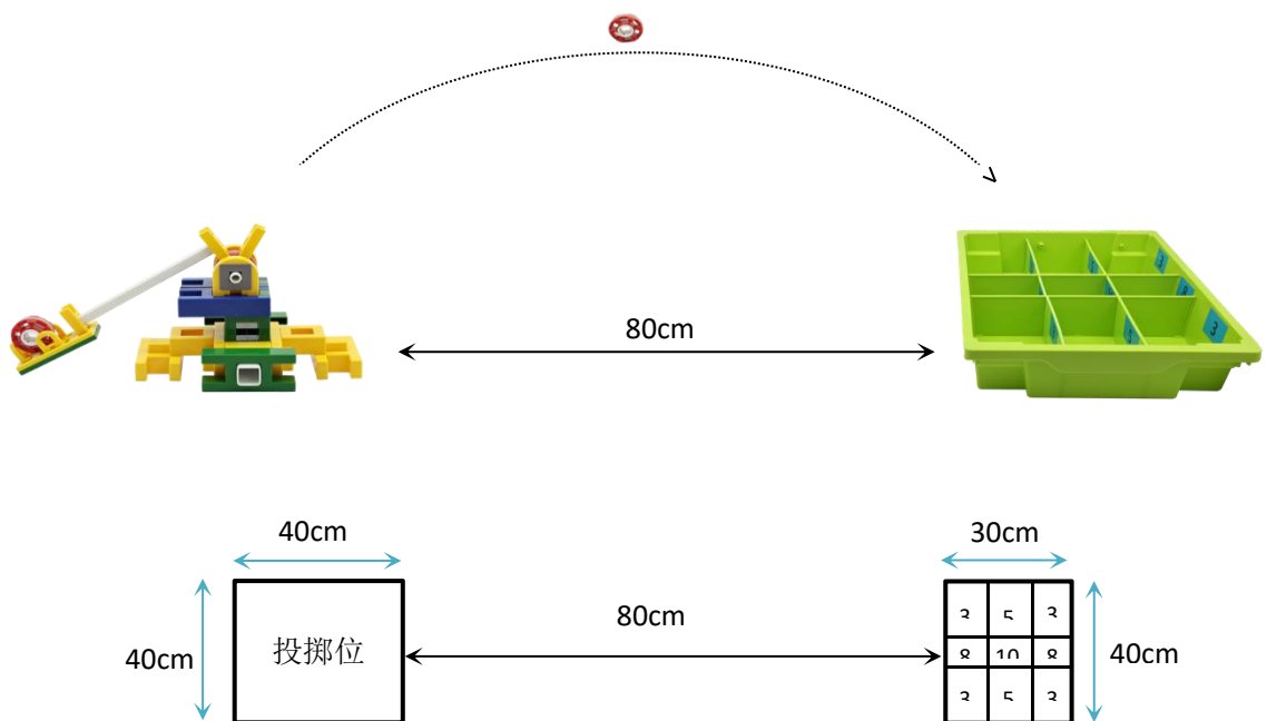
图 1：场地示意图
